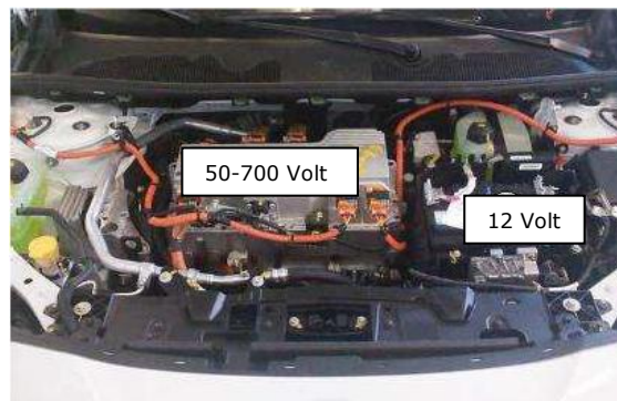
Motorrum på et elkøretøj. De kraftige, strømførende orange ledninger og 12 volt batteriet til højre.
