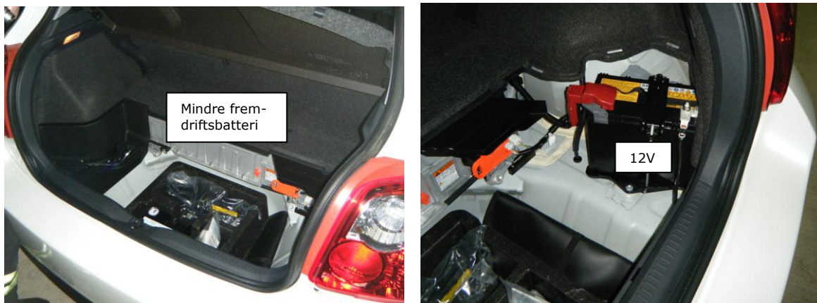
Et eksempel på placeringen af et mindre fremdriftsbatteri i et hybridkøretøj. 12 volts batteriet er i dette tilfælde også placeret i bagagerummet i bagerste højre hjørne.
